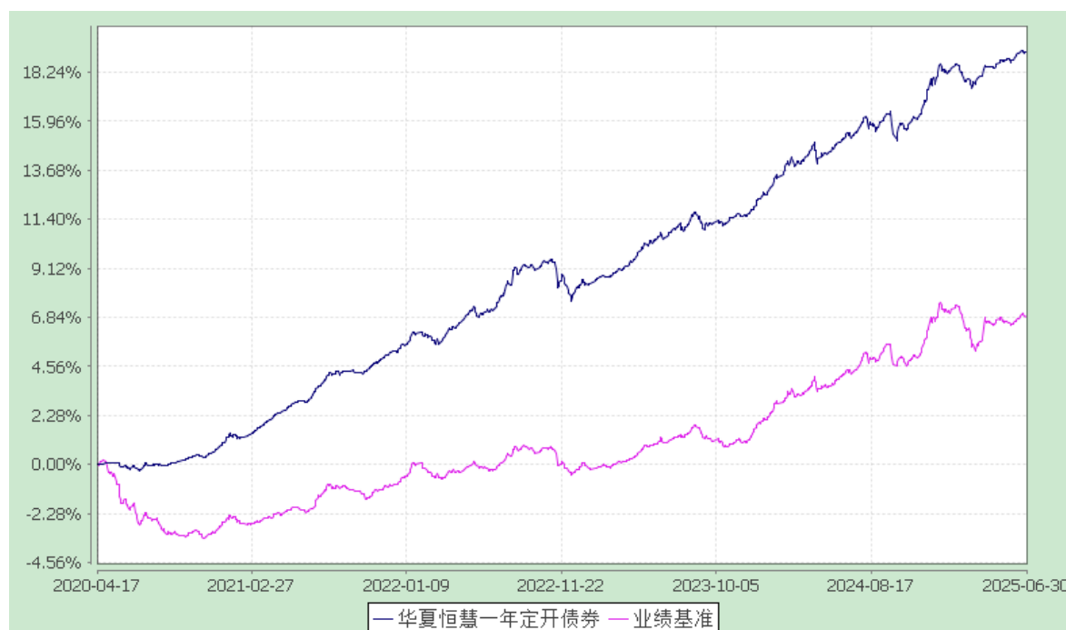
华夏恒慧一年定期开放债券型发起式证券投资基金 累计净值增长率与业绩比较基准收益率的历史走势对比图 (2020年4月17日至2025年6月30日)
